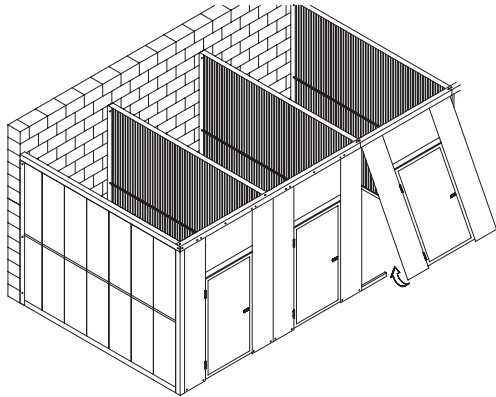
FLUSH DOOR DETAIL
