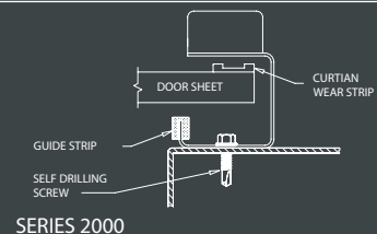
DOOR ENGAGEMENT
